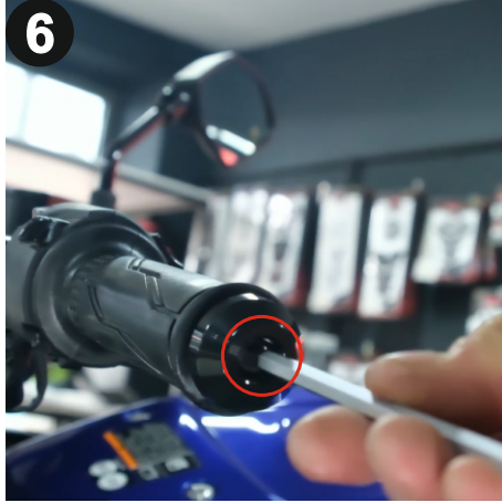
Motosikletinizin gidon topuzunu 5mm alyan kullanarak çıkartınız. (Remove the handlebar end weight using a 5 mm allen.)
