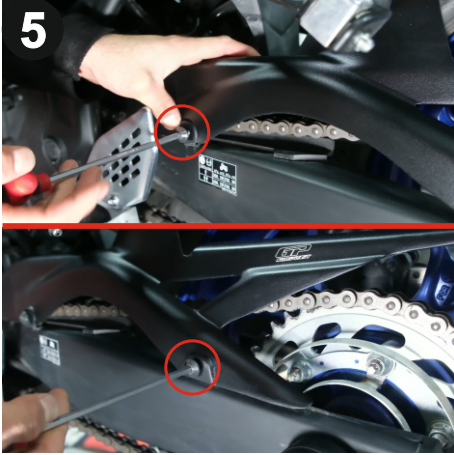
Orijinal vidaları gösterilen şekilde 5mm alyan kullanarak geri monte ediniz. (Reinstall the original bolts as shown using a 5mm allen)
