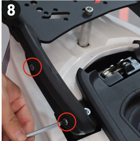
Diğer artçı tutamacını da aynı şekilde monte ediniz. (Mount the other passenger grab handle in the same manner.)
