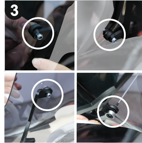
Camı ayaklara konumlandırıp paket içerisinden çıkan cıvata, plastik pul, plastik conta ve somunları 3 alyan ve 8 anahtar yardımıyla sabitleyiniz. (Position the glass onto the feet and secure it using the bolt, plastic washer, plastic gasket, and nut from the package, with the help of a 3 Allen wrench and an 8 wrench.)
