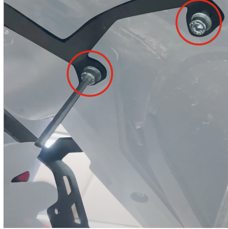
Ürün alt aparatını gösterilen şekilde hizalayın, parçayı 6mm alyan ve contaları kullanarak sabitleyiniz. (Align the product's lower connection accessory as shown, and secure the part using a 6mm Allen key and seals)
